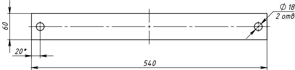
Поз.3 (Полухомут) развертка
