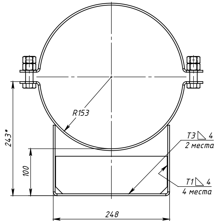
Поз.3 (Полухомут)
