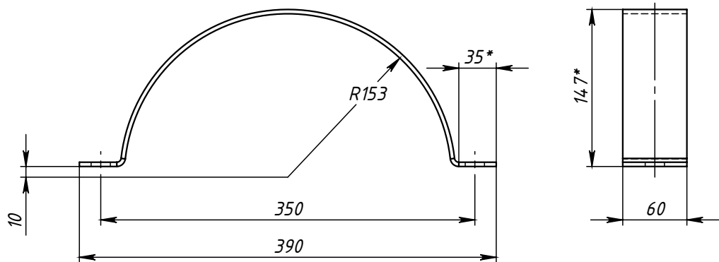
Поз.3 (Полухомут)
